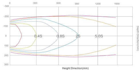
数显直流离子风机JN100D除电时间特性图
