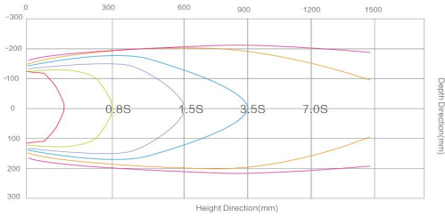
数显交流离子风机JN100A除电时间特性图
